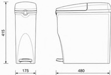
DIBUJO TÉCNICO (mm)
