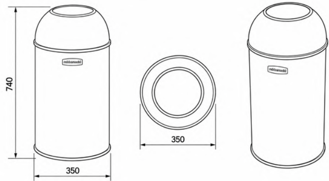
DIBUJO TÉCNICO (mm)
