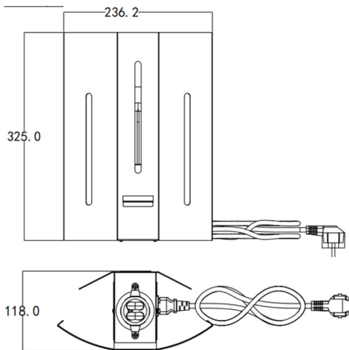
DIBUJO TÉCNICO
